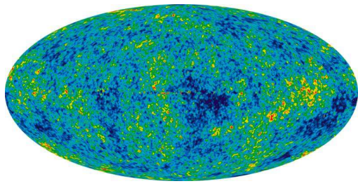
საწყისი არაერთგვაროვნებები: გალაქტიკების ჩანასახები
